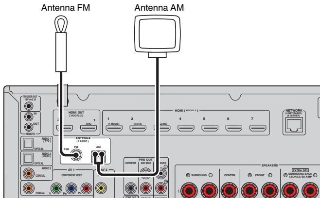
Unità (retro)
