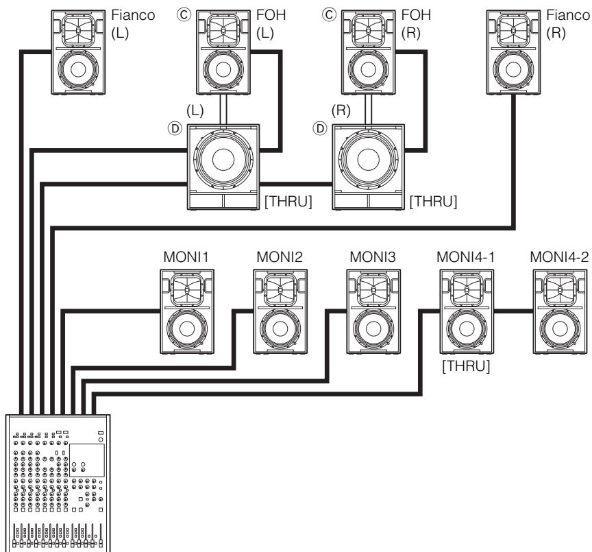
Mixer analogico
