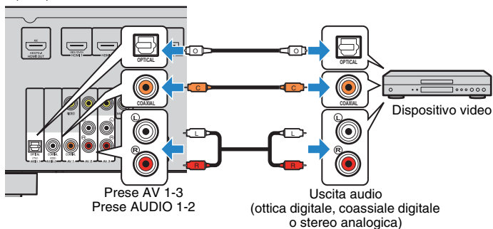
Unità (retro)
